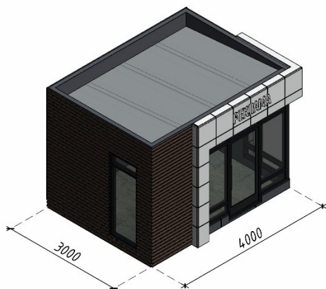
НТО 4х3м
