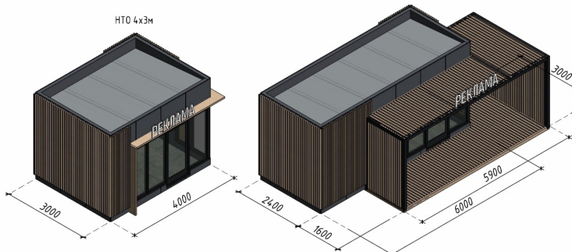
НТО 6х2,4м с размещением навесом
