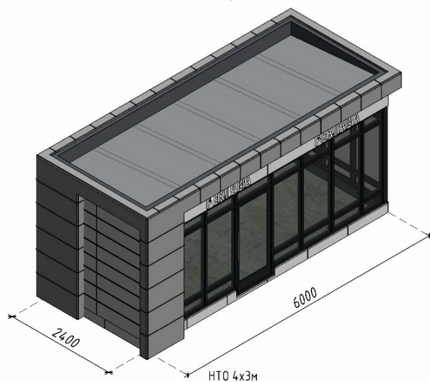
НТО 6х2,4м
