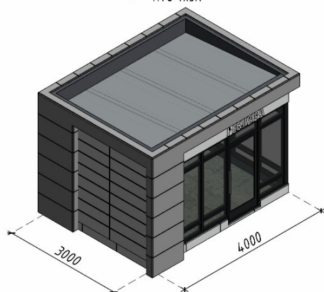
НТО 4х3м
