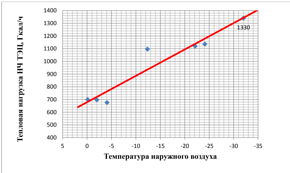
Рис. 1.1. Динамика тепловой нагрузки НЧ ТЭЦ в зависимости от температуры наружного воздуха
